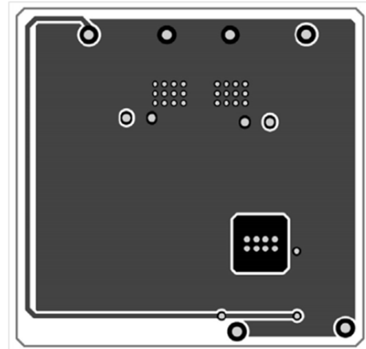
Fig. 17 Bottom Layer
