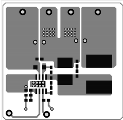
Fig. 16 Top Layer
